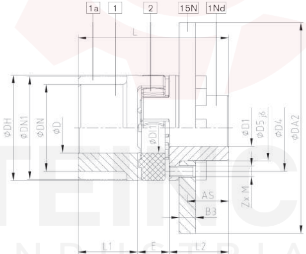
Bremsscheibe Bauart SBAN
