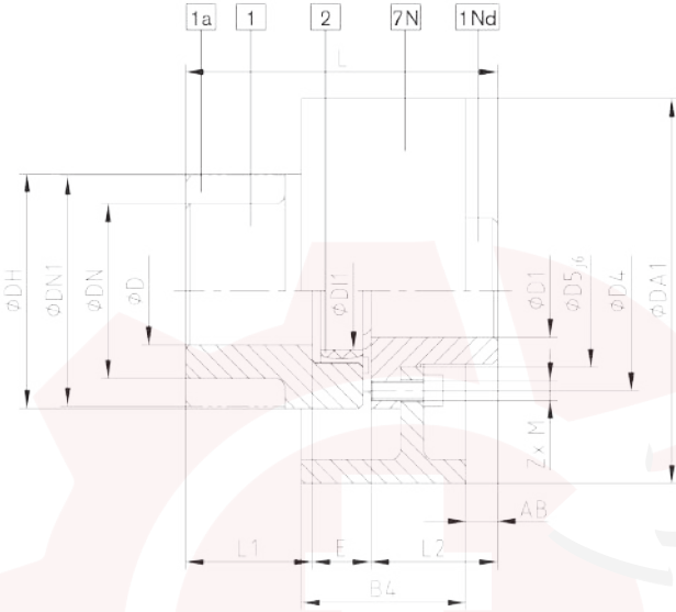
Bremstrommel Bauart BTAN
